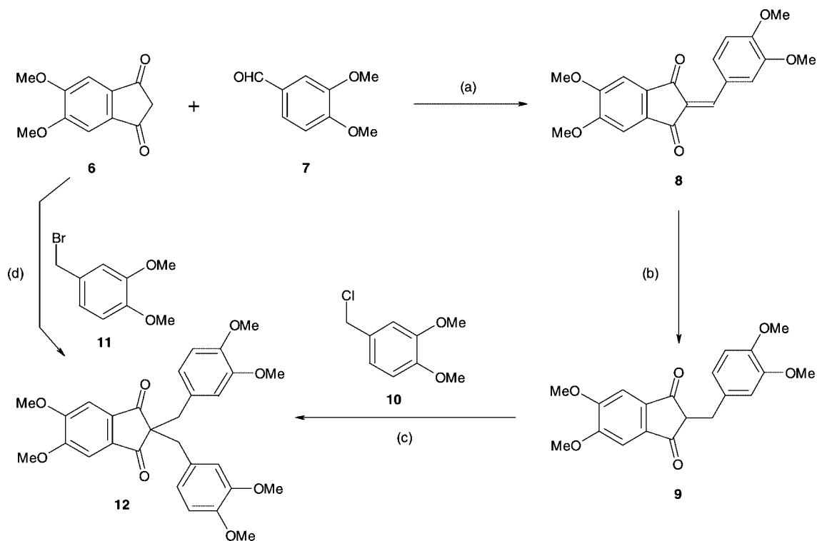
Scheme 2. (a) AcOH, \Delta , 2 h, 88%; (b) NaBH 4 , pyridine, 60 °C, 20 min, 84%; (c) KF/celite 545, acetonitrile, 75 °C, 3 h, 79%; (d) KF/celite 545, acetonitrile, 75 °C, 4 h, 38%.
