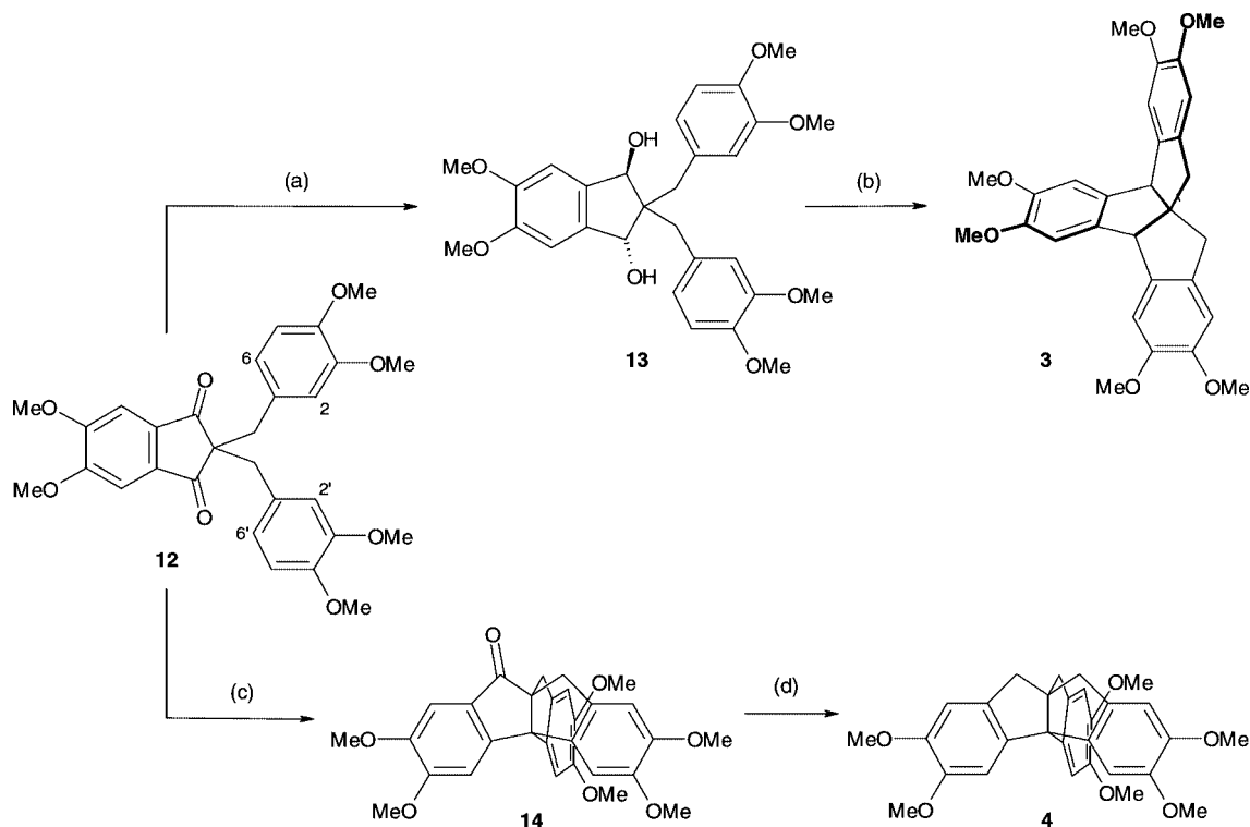
Scheme 3. (a) \text{LiAlH}_4 , THF, \Delta , 4 h, 73%; (b) \text{H}_3\text{PO}_4 (85%), chlorobenzene, \Delta , 1 h, 66%; (c) \text{H}_3\text{PO}_4 (85%), toluene, \Delta , 7 h, 73%; (d) \text{NaBH}_4 , \text{CF}_3\text{COOH}/\text{CH}_2\text{Cl}_2 , 20^\circ\text{C} , 48 h, 68%.
